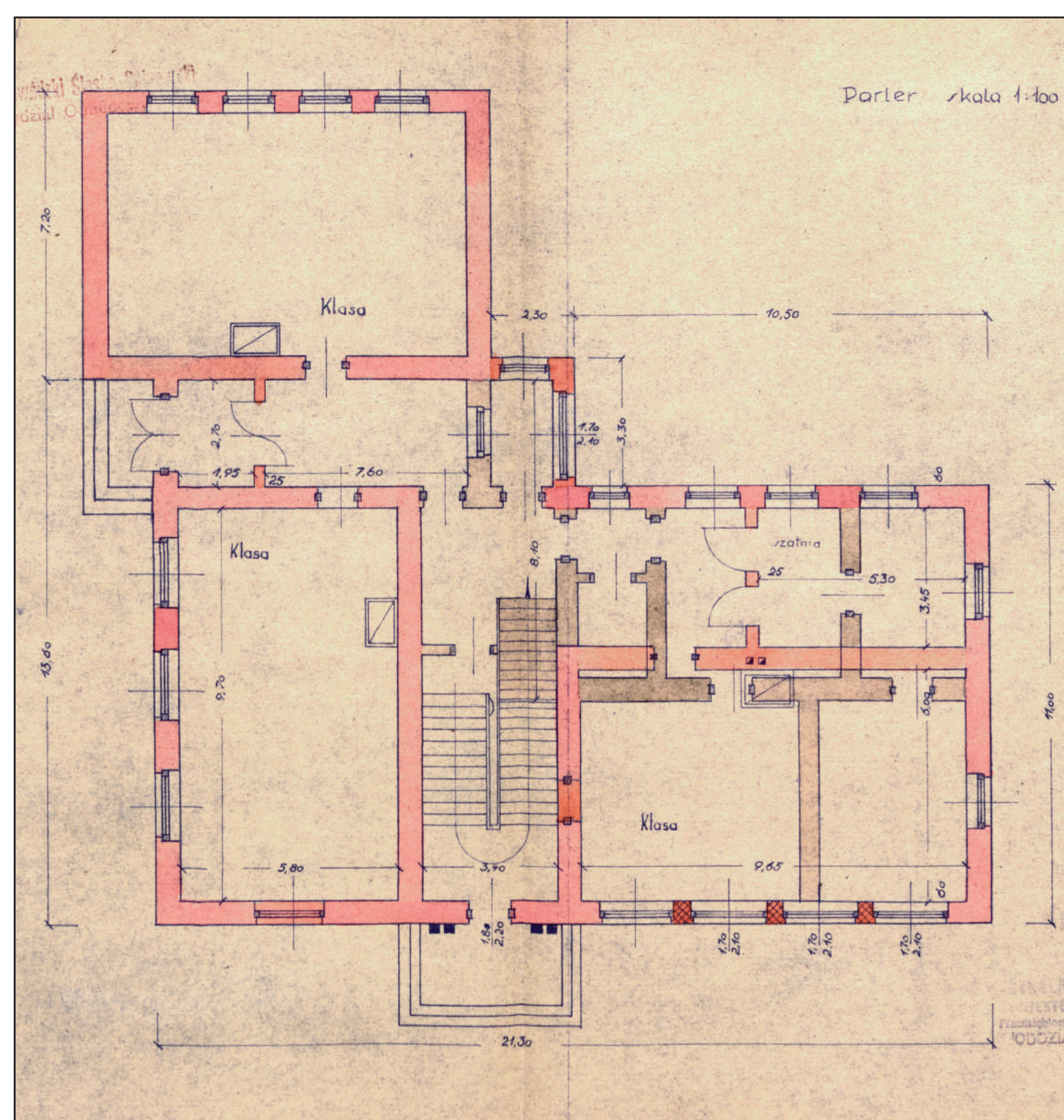
Projekt przebudowy budynku Szkoły nr 2 w Wójtowej Wsi - parter z 1947 r.
